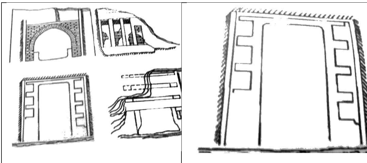
Расми 28 Нақшаи хумдони хиштпазии Вошгирд (аск аз Д. Довуди, манба Археологические работы в Таджикистане . Вып.30. – С.205-223)
