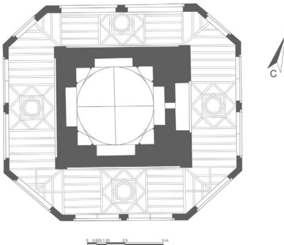
Расми 36. Тарҳи меъмории мақбараи Мавлоно Тоҷиддин (акс аз бойгонии шуъбаи бостониносии Институти таърих, бостониносии ва мардуминосии)
